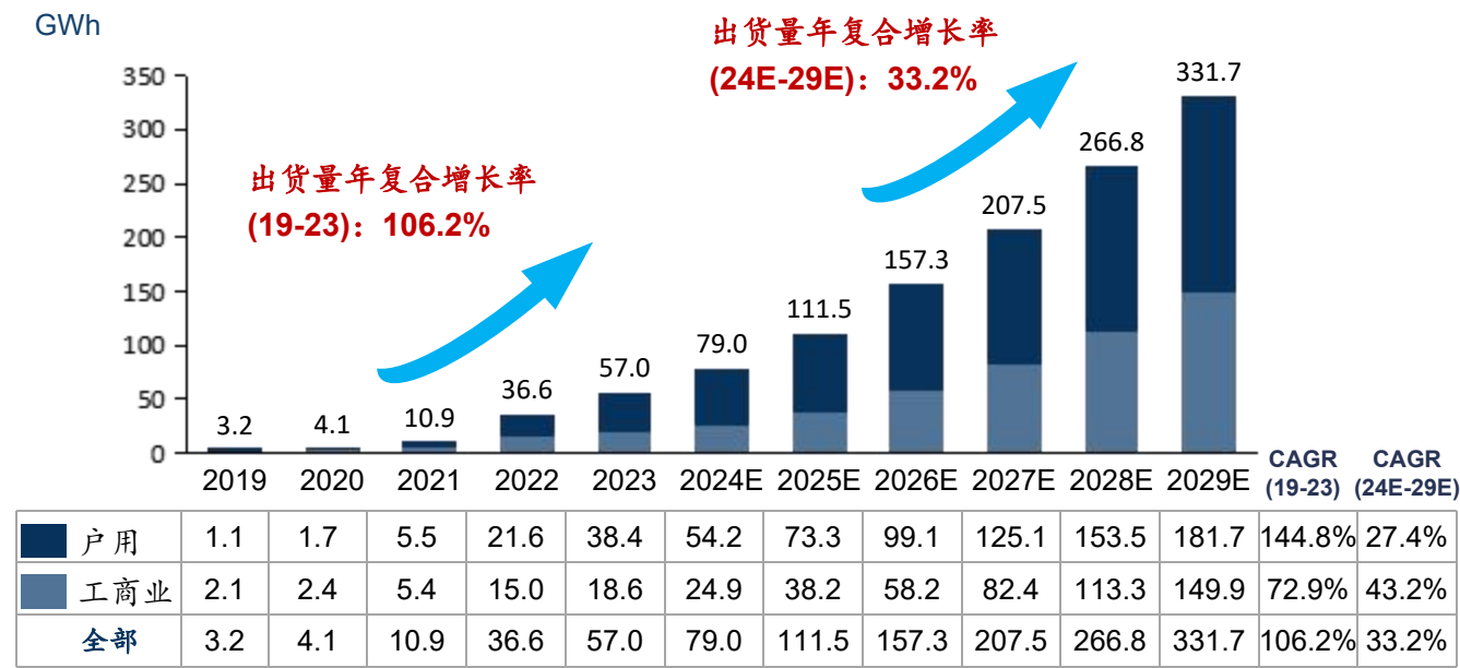
分布式储能系统年出货量（按下游应用划分），全球，2019-2029E
